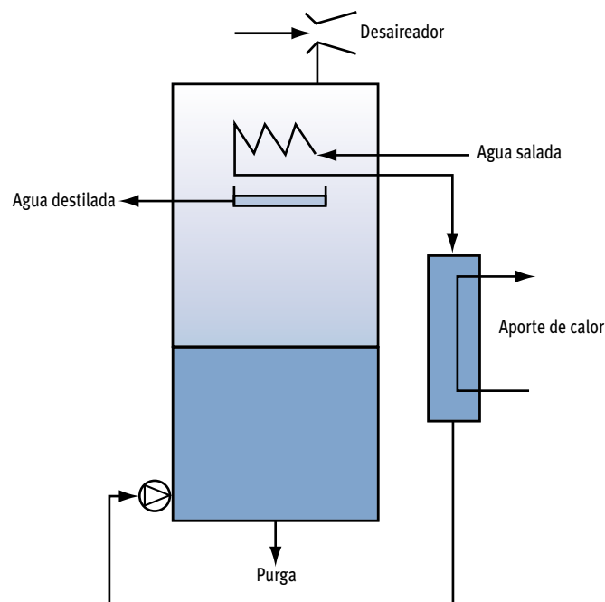
Figura 15. Sistema de destilación por expansión brusca de líquido saturado
