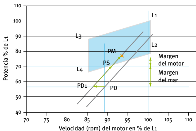
Figura 10. Punto de diseño del propulsor del buque en relación al paralelogramo de diseño de un motor diésel
