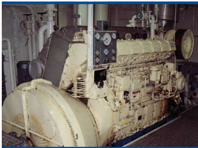
Motor diésel turboalimentado
