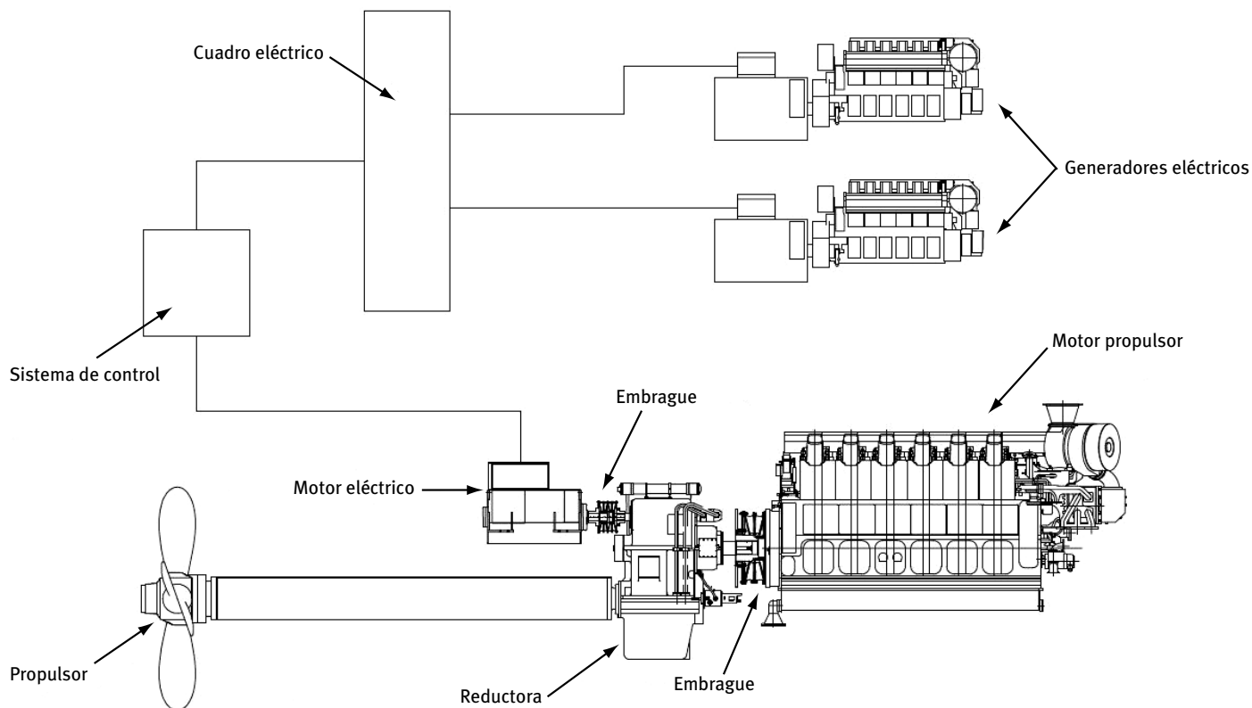
Figura 16. Esquema de un sistema de propulsión diésel-eléctrico.
