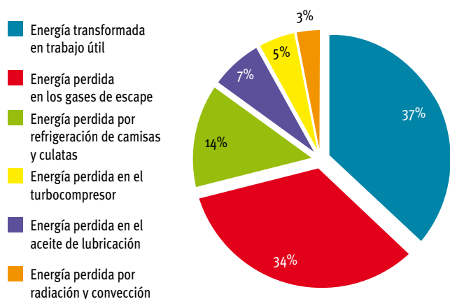
Figura 14. Balance térmico de un motor diésel de cuatro tiempos sobrealimentado
