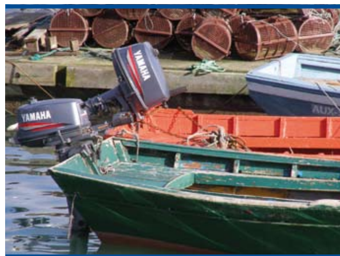
Motor fuera borda de dos tiempos convencional
